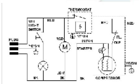
Схема электрическая принципиальная «BIRUSA V032E»
